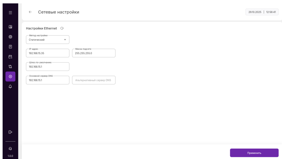
Рисунок 57 — Сетевые настройки
