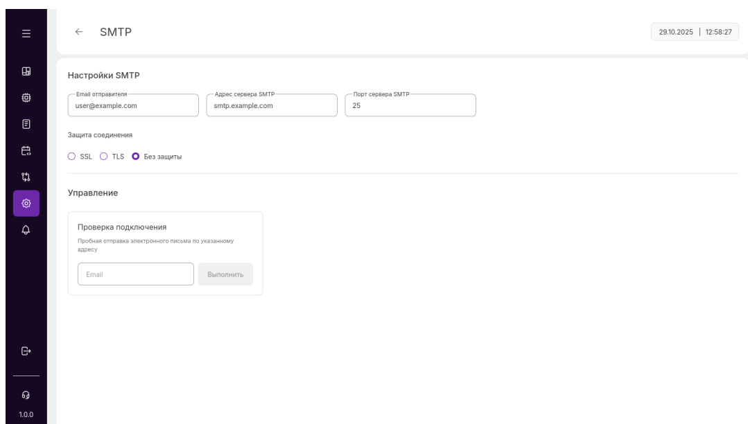
Рисунок 59 — Настройки SMTP
