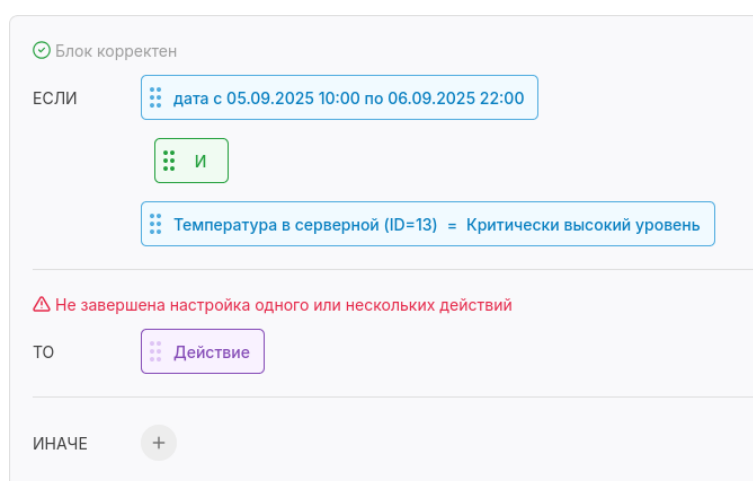
Рисунок 46 — Отображение условия
