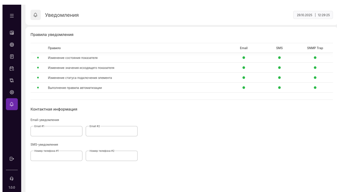
Рисунок 50 – Раздел "Уведомления"
