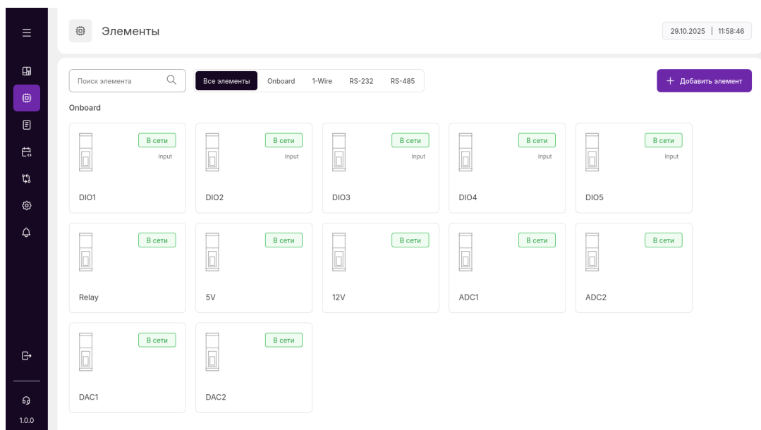
Рисунок 19 – Раздел "Элементы"
