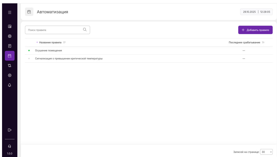
Рисунок 34 — Раздел "Автоматизация"
